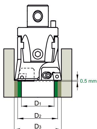
Barenatura sfalsata
