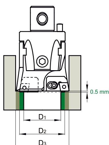
Cartuccia sfalsata
